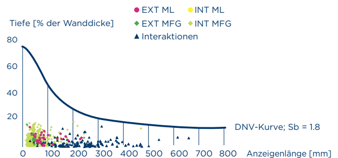
Molchanzeigtiefe und -länge mit DNV-Grenzkurve
