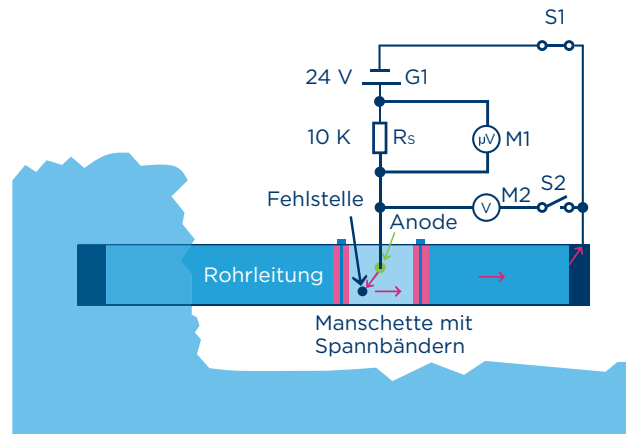
Elektrolytische Porenprüfung (OGE-Eigenentwicklung)
